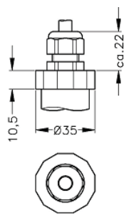
кабельный ввод для кабеля с воздушной трубкой (IP 67)
