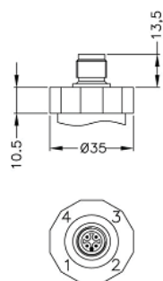
разъём M12x1, 4-конт. (IP 67)
