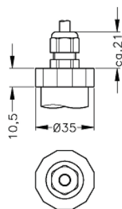
кабельный ввод для кабеля без воздушной трубки (IP 67)
