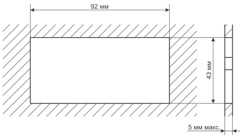
Рисунок 2.2. Допускаемое отверстие для монтажа индикатора.
