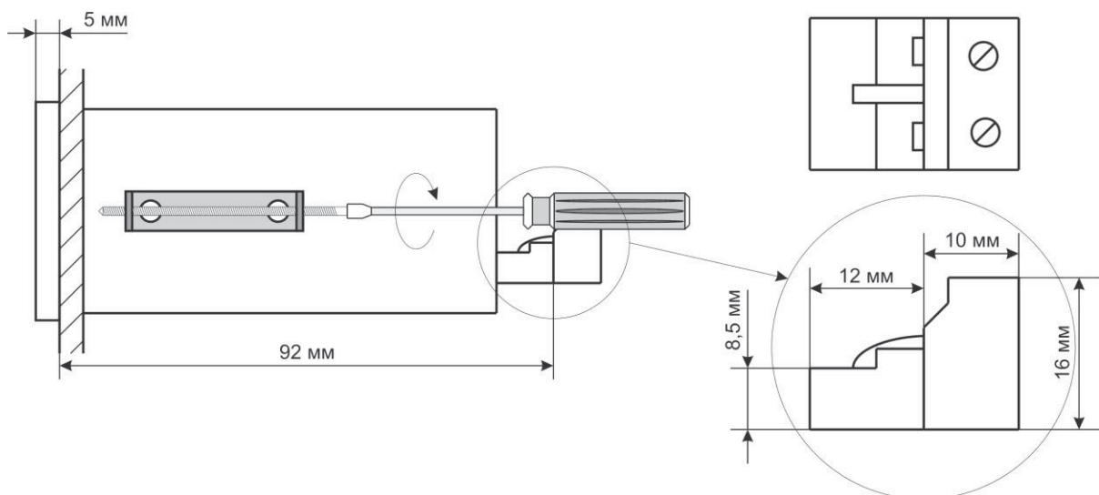
Рисунок 2.3. Установка фиксирующих зажимов. Размеры клеммной колодки.
