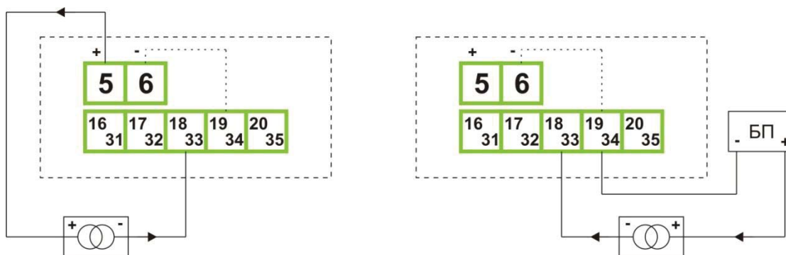
Рисунок 2.9. Схемы включения преобразователя 4...20 мА / 2-х пров. Слева – с использованием встроенного источника питания, справа – с использованием внешнего источника питания.
