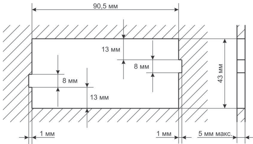
Рисунок 2.1. Рекомендованное отверстие для монтажа индикатора.
