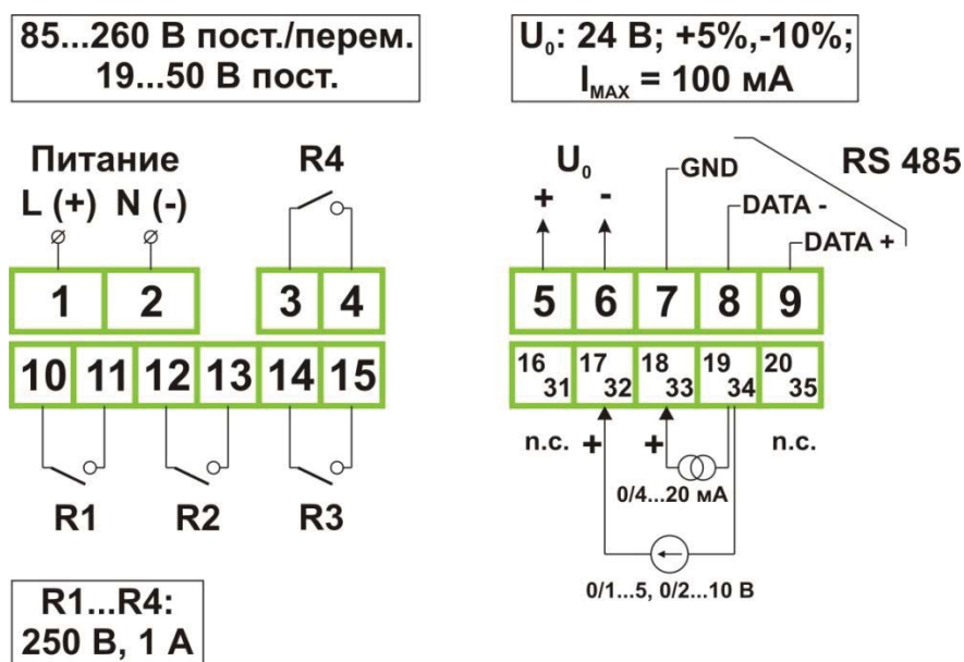
Рисунок 2.6. Обозначение контактов (тип реле – “сухой контакт”, исполнение без активного токового выходного сигнала).
