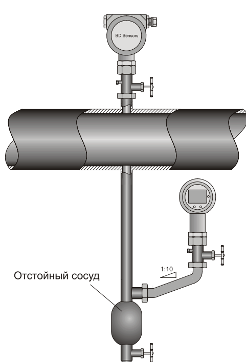
Рисунок 12. Монтаж датчика
