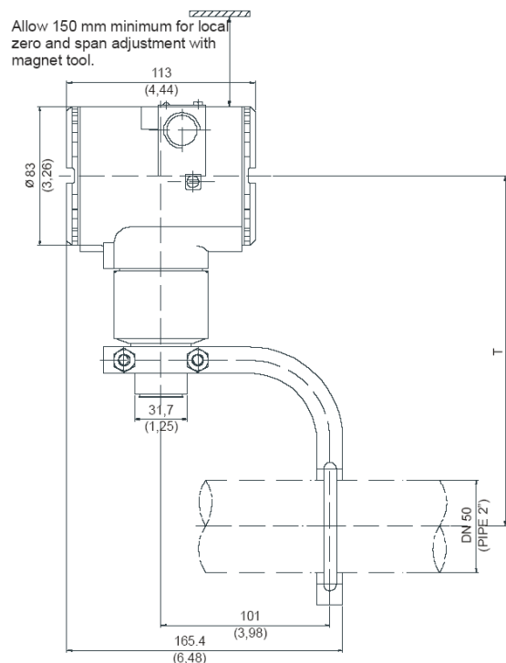
Рисунок Б.1 – Датчик НМР 331-А-S.
